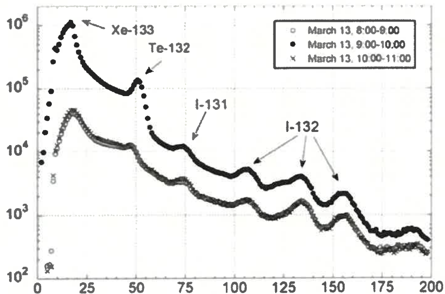
大熊町大野のモニタリングポスト 2011年3月13日8:00-11:00の波高分布図
