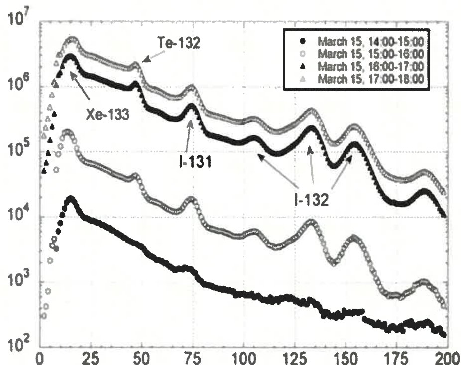
福島市紅葉山のモニタリングポスト 3月15日の14:00-18:00の波高分布図
