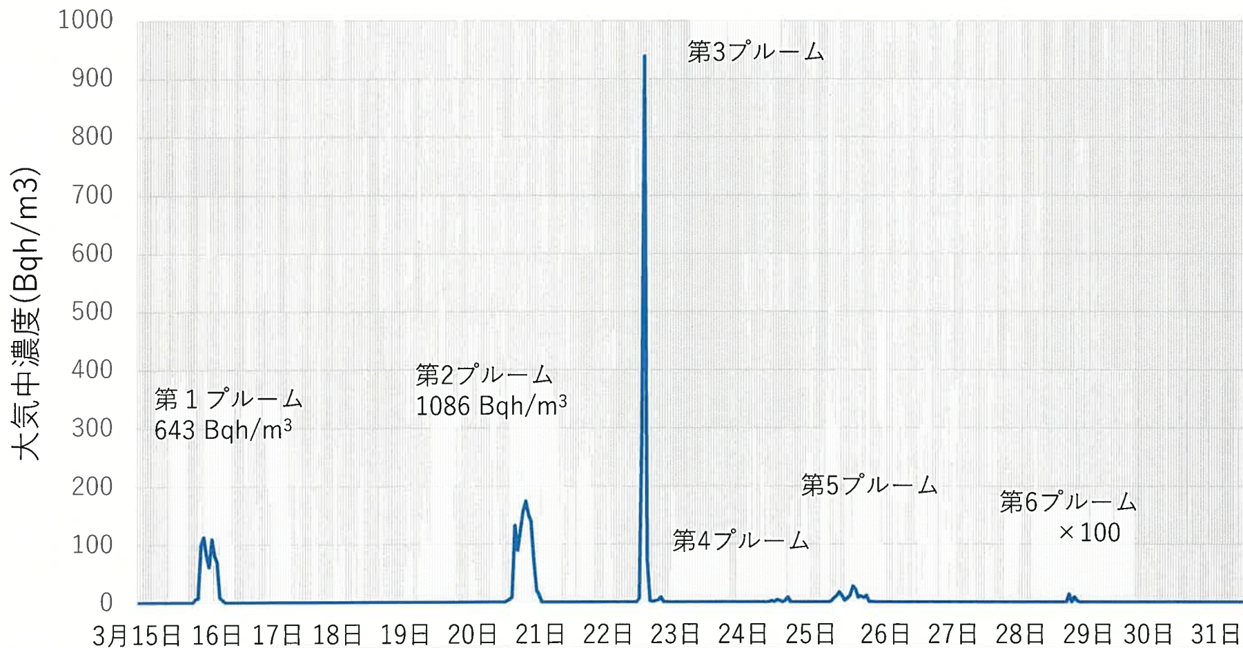
ATDMが示す6つのプルームの 131 Iの大気中濃度
